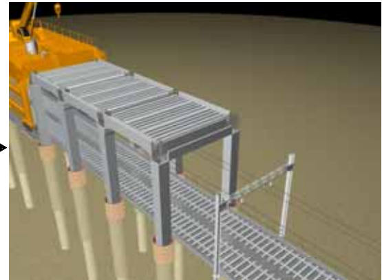
ハーフプレキャストスラブの架設
