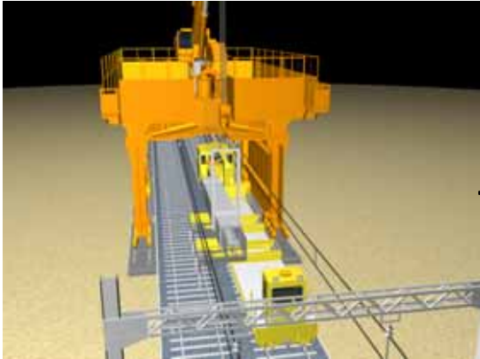
ハーフプレキャスト部材の運搬
