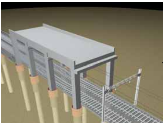
梁，スラブの場所打ちコンクリートを打設後，完成
